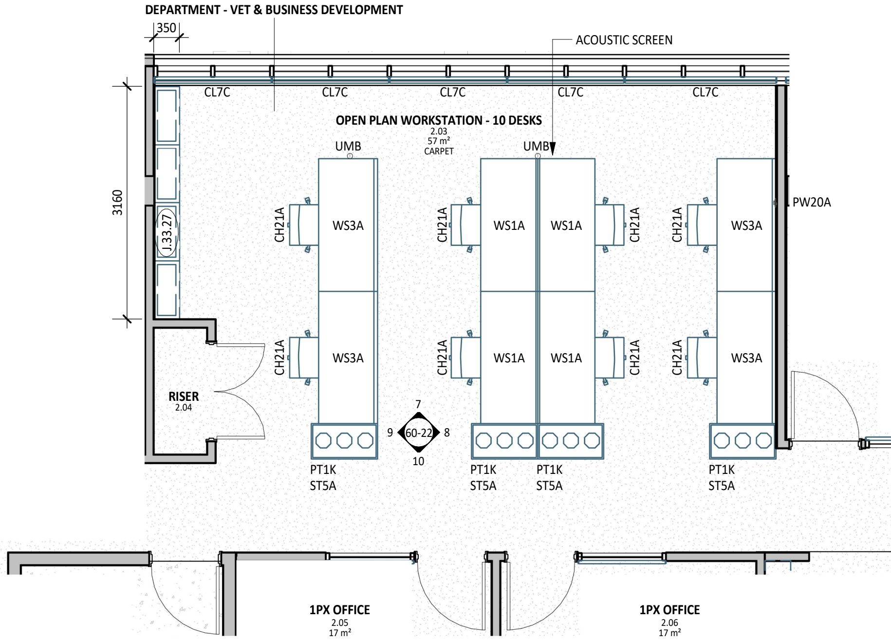
6 PLAN DETAIL 1 : 50
