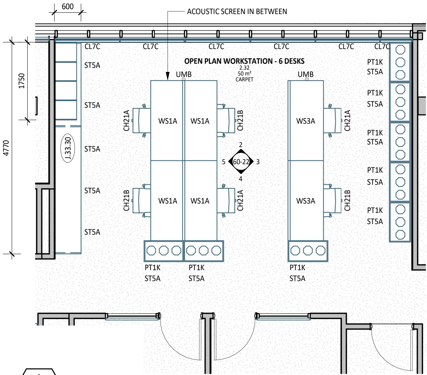
1 PLAN DETAIL 1 : 50
